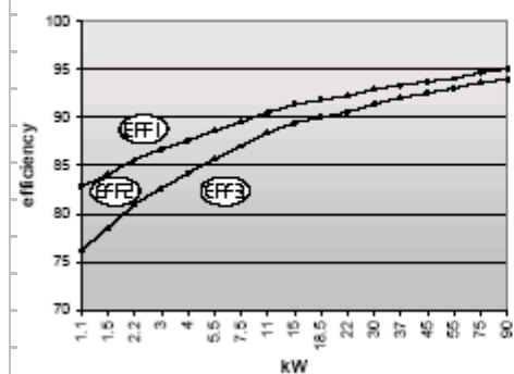
2 - pole
